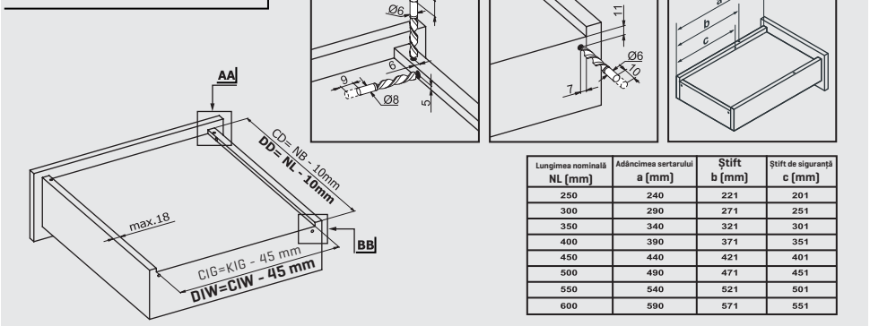
Realizarea găurilor pentru Pin-Fix (Fixare cu pin)
