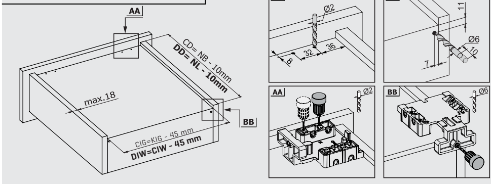
Realizarea găurilor pentru Lock-Fix (Fixare cu conectori)
