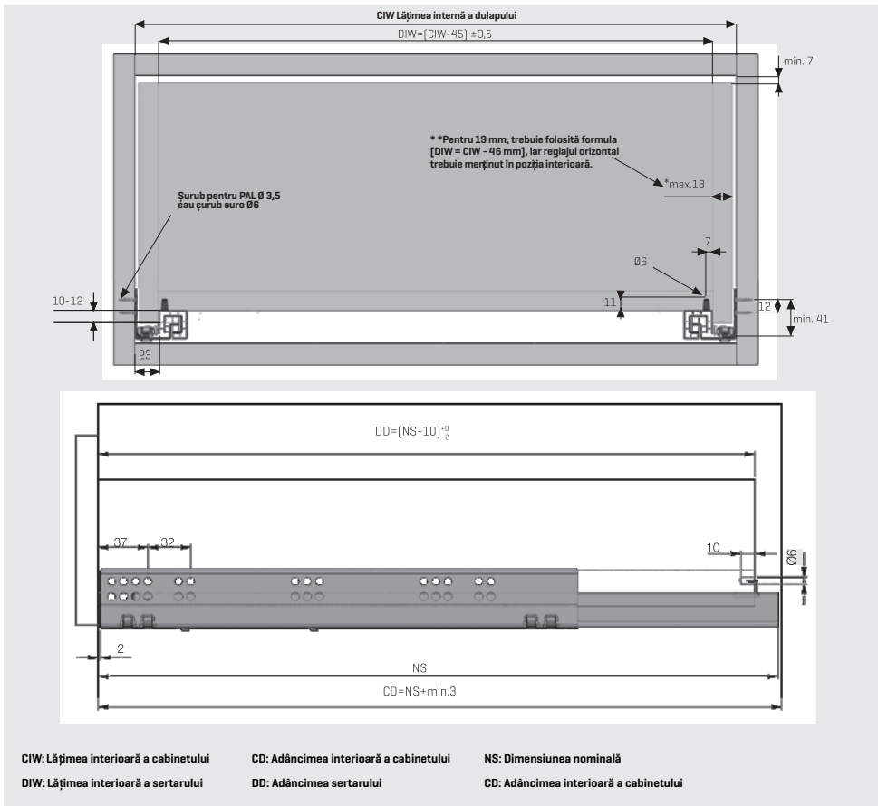
Realizarea găurilor pentru Lock-Fix (Fixare cu conectori)
